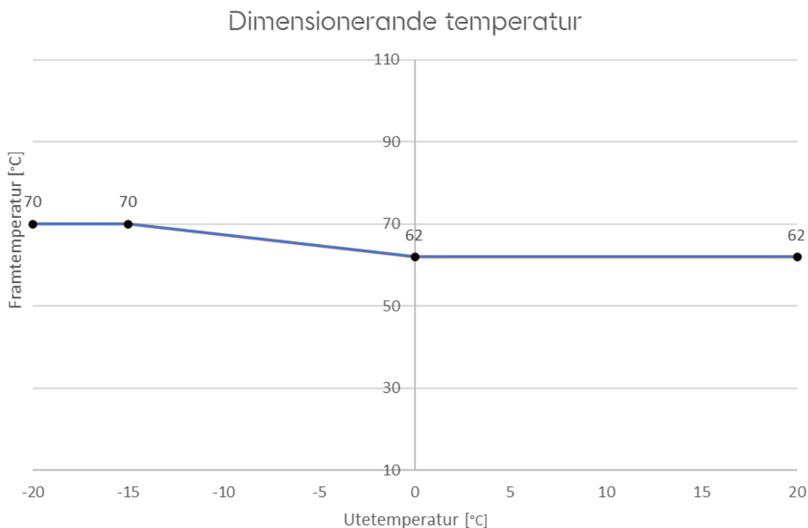
Figur 2. Dimensionerande drifttemperatur framledning fjärrvärme.
