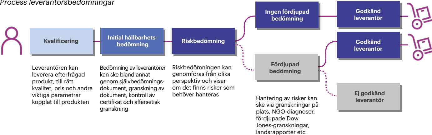
Figur 3. Process leverantörsbedömningar
