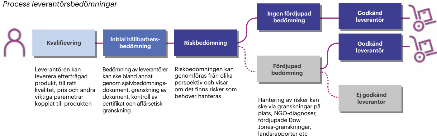
Figur 3. Process leverantörsbedömningar
