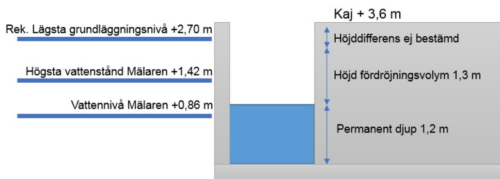
Figur 15 - Skiss över placering av dammsystem väst i förhållande till Mälarens medevattennivå. Nivåskillnader i bild är inte skalenliga.
