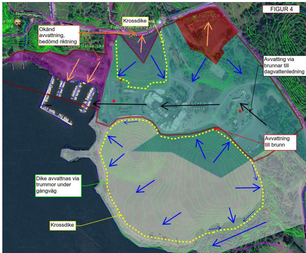
Figur 4 – Befintligt område och översiktliga avvattningsvägar. Blå pilar avser avrinningsriktningar från mark och svarta pilar ledningsbunden avrinning. Orangea pilar markerar bedömd avrinningsriktning från områden med okända dagvattenanläggningar. Röda punkter markerar dagvattenbrunnar.
