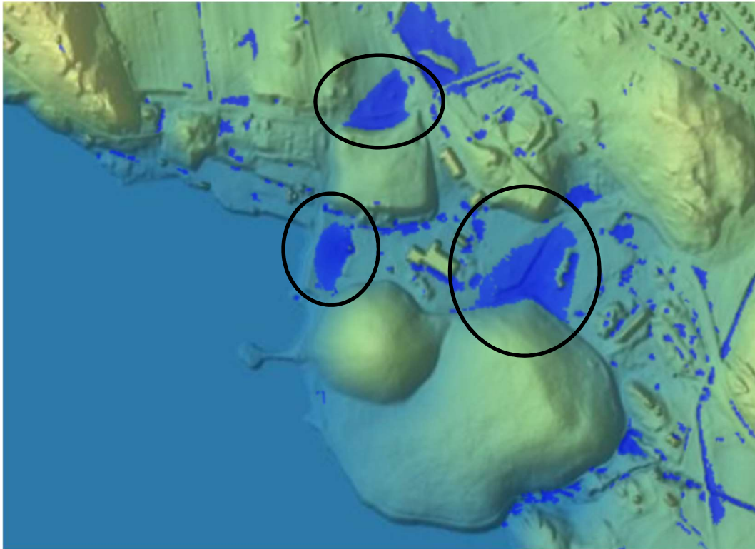
Figur 18 – Översvämningssituation för planområdets nuvarande förhållanden framtagen i Scalgo. Områden med risk för översvämning vid skyfall inom och i anslutning till planområdet är markerade med svarta ovaler.
