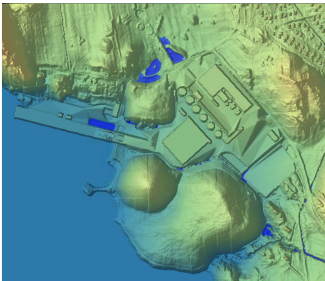
Figur 20 - Översvämningssituation för framtida situation enligt planförslaget framtagen i Scalgo. Endast områden med stående vatten djupare än 50 cm redovisas.
