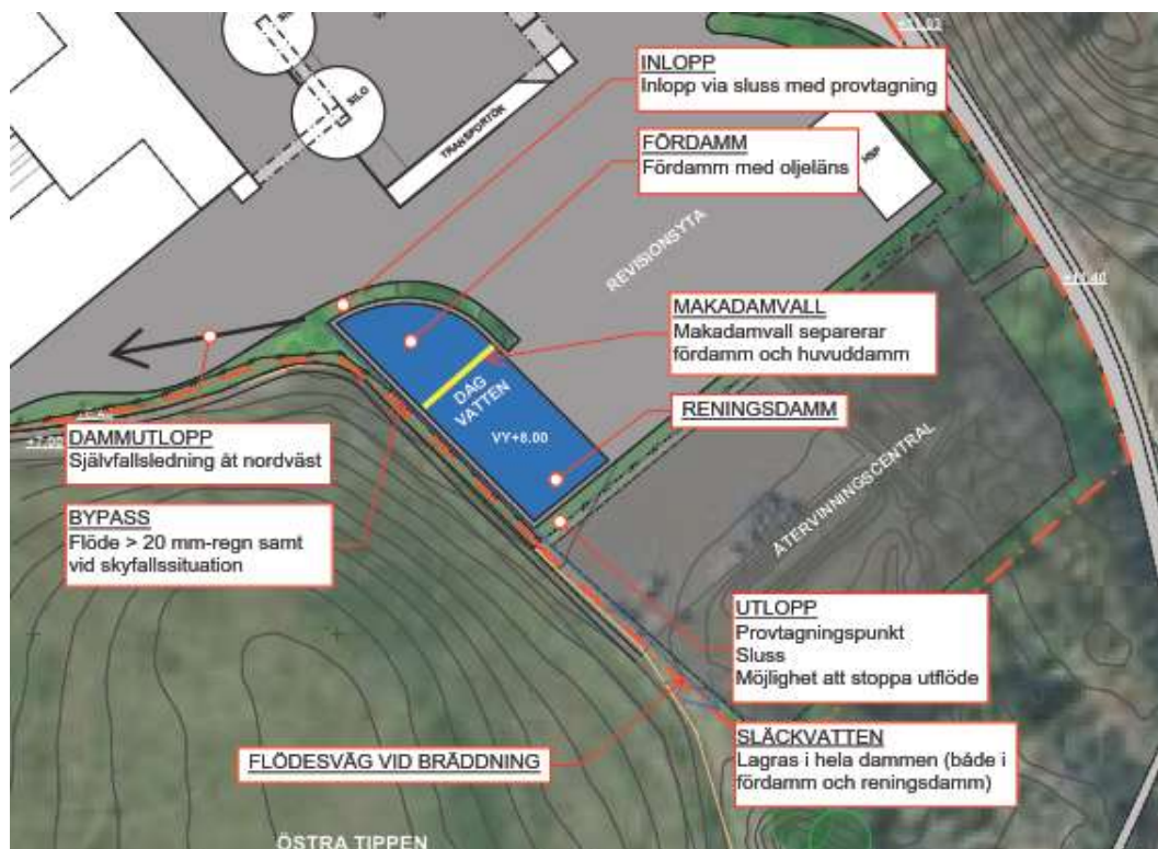
Figur 16 - Utformning dammsystem öst.
