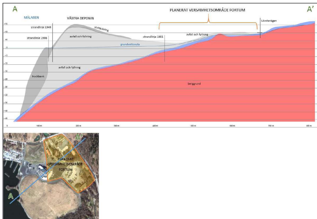
Figur 5 – Tvärsektion över marklager för Lövstatippen. Bild: Geosigma 2017.
