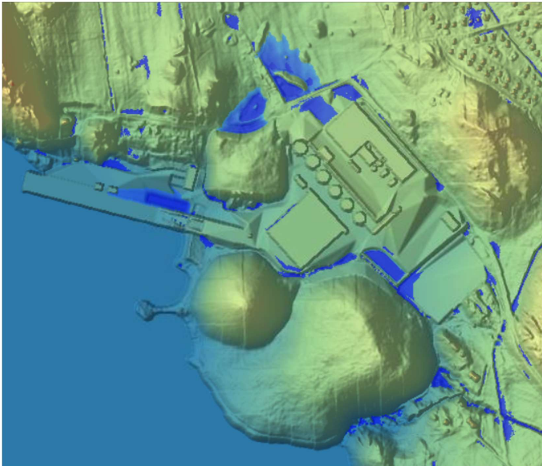
Figur 19 – Översvämningssituation för framtida situation enligt planförslaget framtagna i Scalgo. Blå färg markerar stående vatten. Figuren redovisar alla vattensamlingar oavsett djup.
