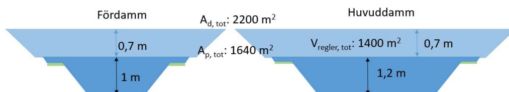
Figur 11 - Dammsystem öst med fördamm och huvuddamm.
