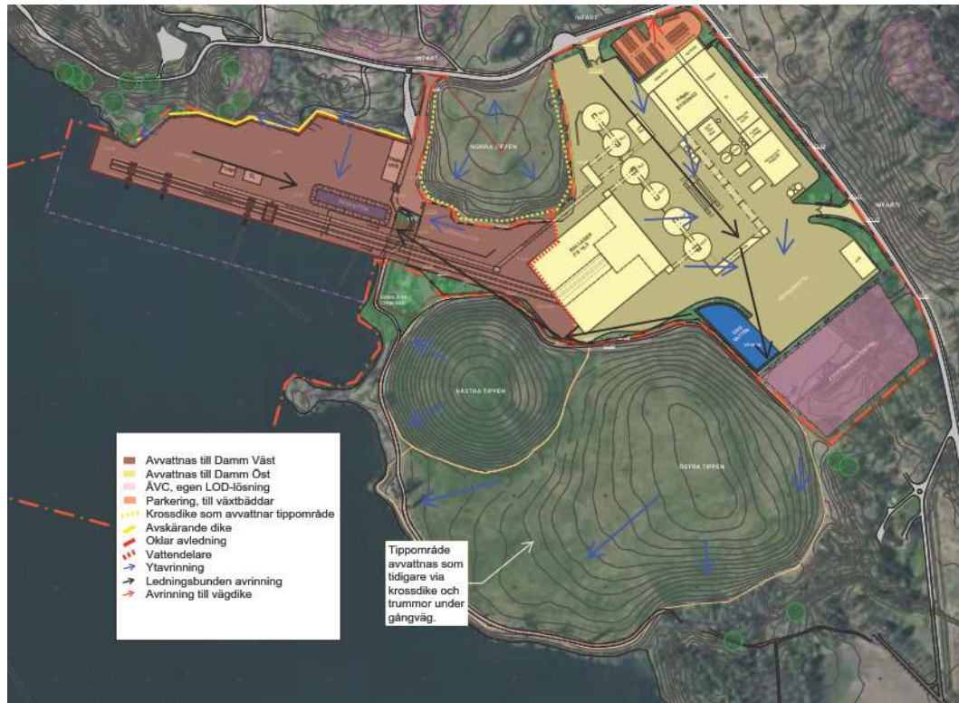
Figur 13 – Föreslagna avvattningsvägar för kommande exploatering vid normal drift.
