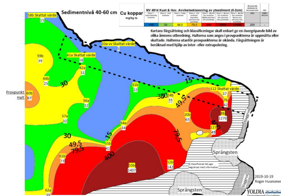
Figur 7: Koppar 40-60 cm.
