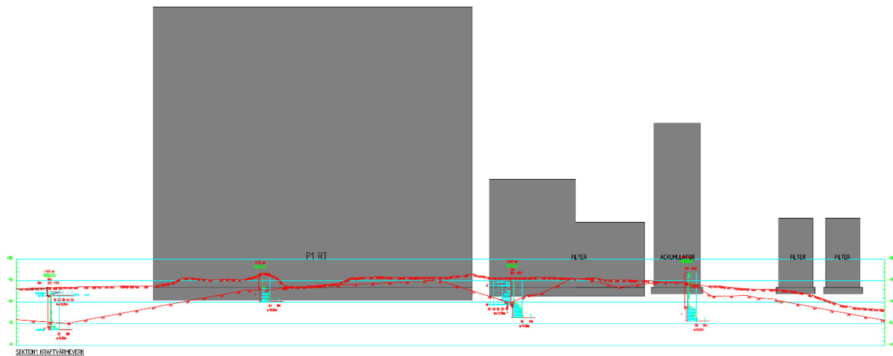
Figur 14. Sektion1 Kraftvärmeverk redovisar anläggningen i förhållande till berg och markytan. För läge i plan se figur 13.
