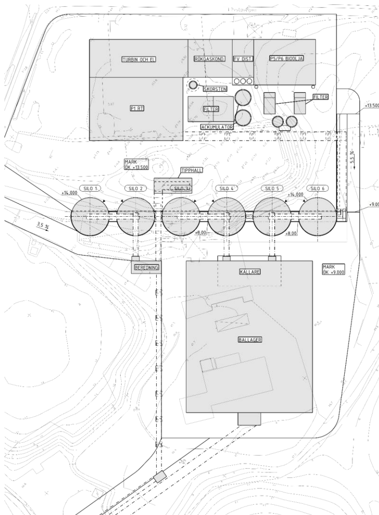
Figur 3. Planerad anläggning och höjdsättning, K05 (2018-10-09, WSP).
