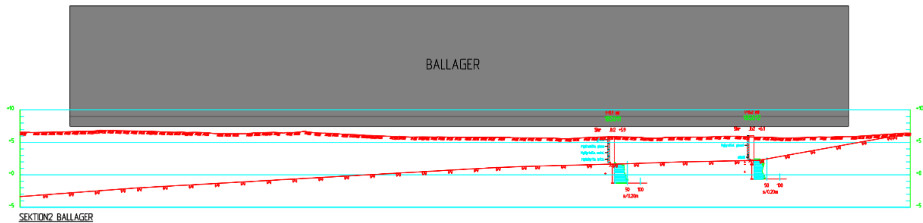
Figur 25. Sektion2 BALLAGER redovisar anläggningen i förhållande till berg och mark. För läge i plan se figur 23.
