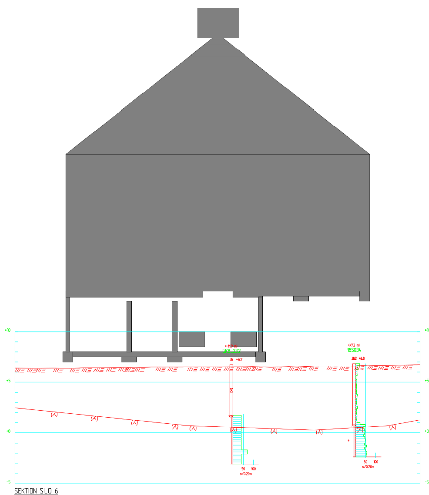
Figur 22. Tvärsnitt av Silo 6. För läge i plan se figur 16.
