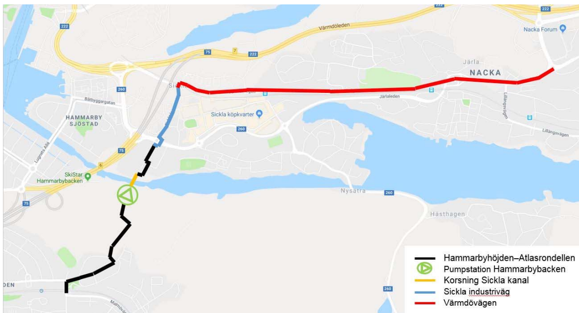
De fem etapperna i en ny huvudledning till Nacka.
